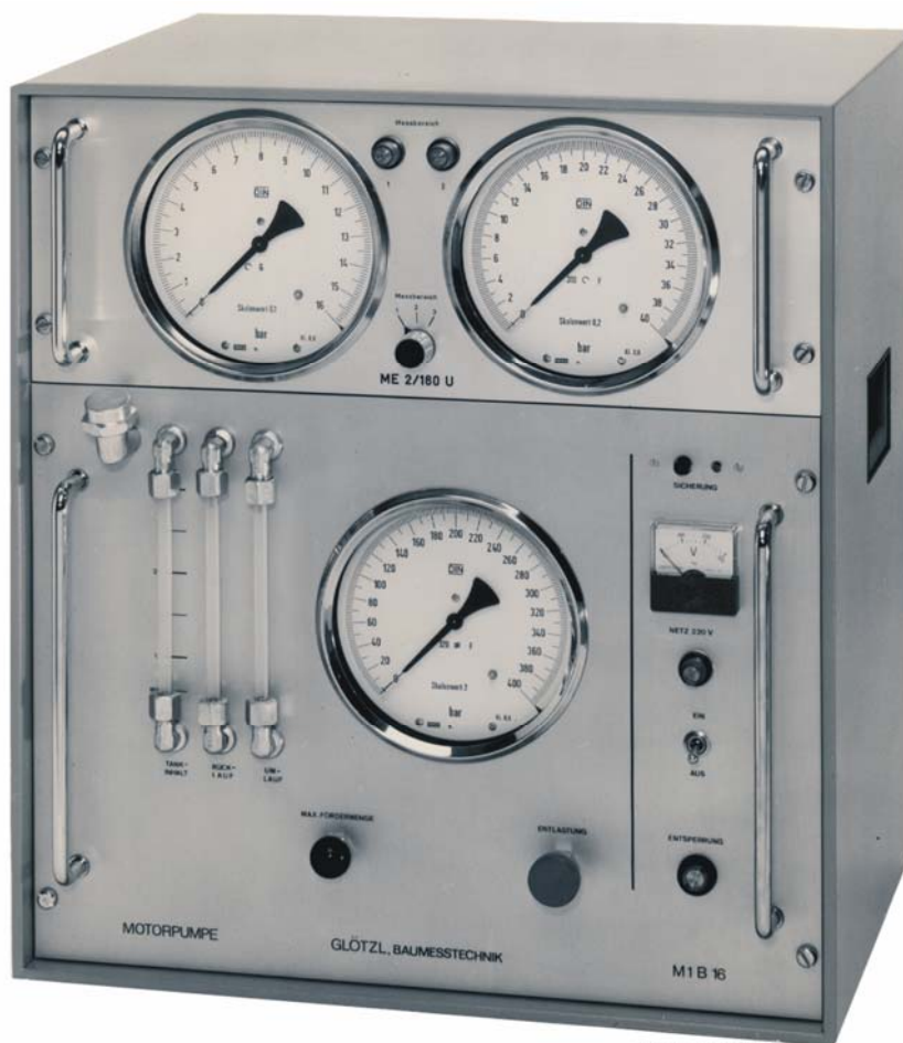
Abb.: Zusatzeinheit, ME2/160 U mit Motorpumpe
